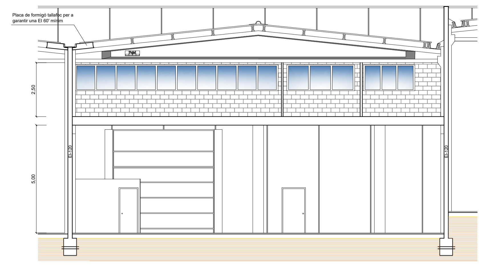
SECCIÓ A-A'
