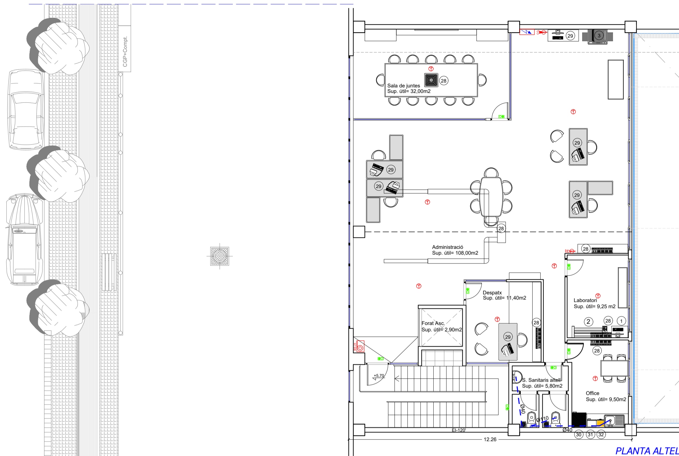
PLANTA ALTELL
