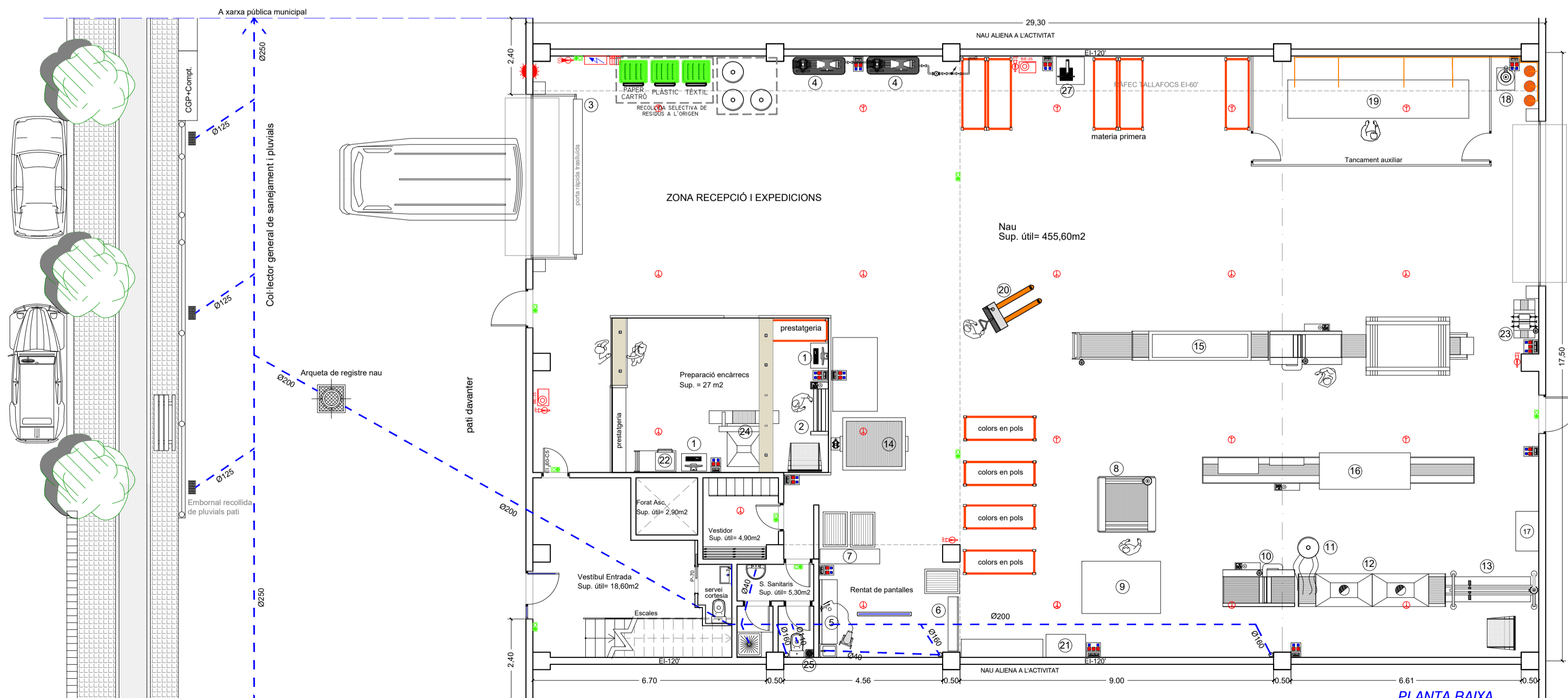
PLANTA BAIXA
