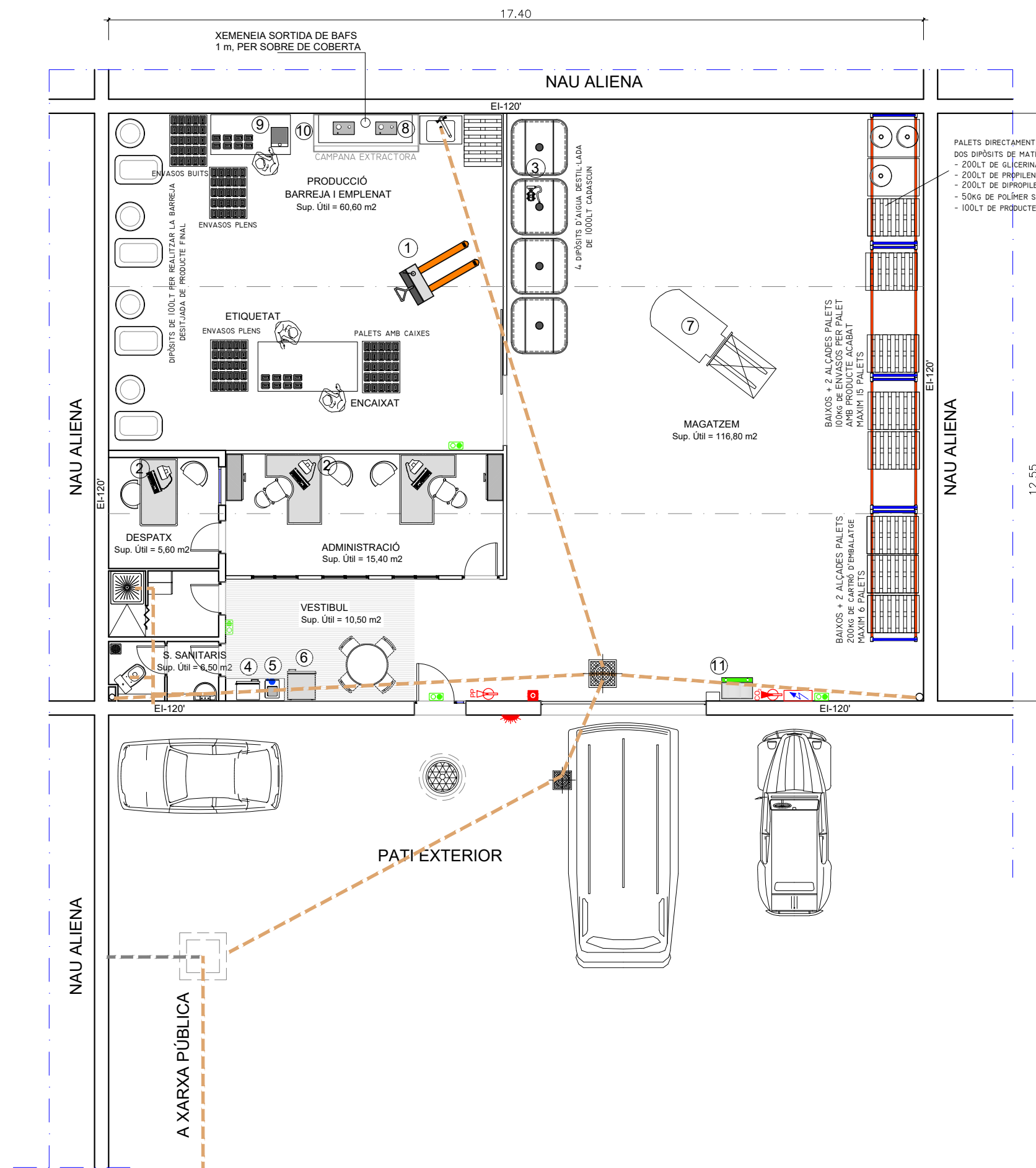
PLANTA BAIXA Sup. Útil total = 215,40 m 2 Sup. construïda total = 230,10 m 2
