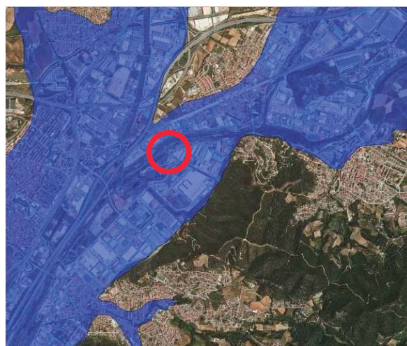
Imatge 7. Masses subterrànies (Font: Visor ACA)
