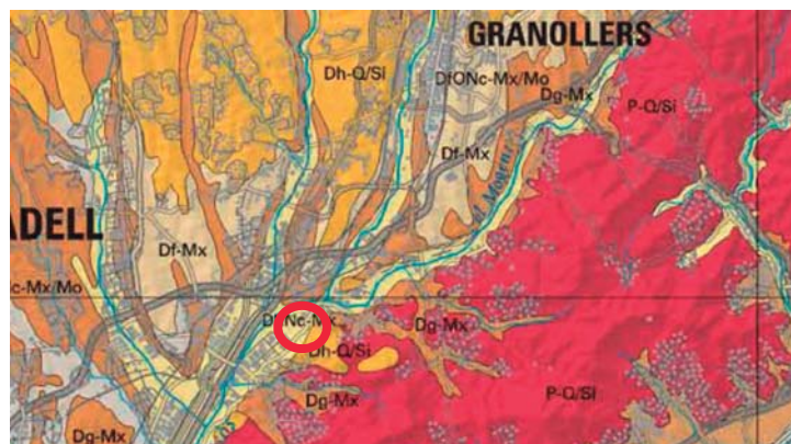
Imatge 4. Mapa de grups litològics (Font: ICGC)
