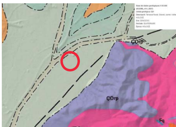
Imatge 3. Dades geològiques (Font: www.betaportal.icgc.cat )
