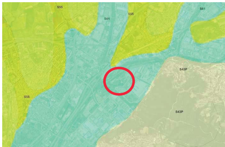
Imatge 4. Unitat cartogràfica (S61) i classificació del sòl (Font: ICGC)
