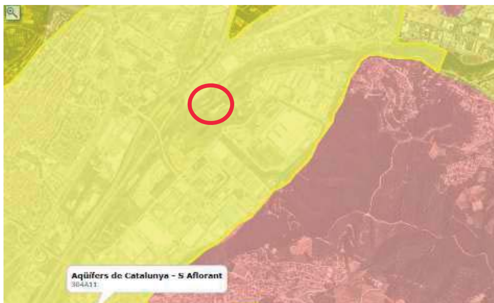
Imatge 8. Aquífers de Catalunya (Font: visor ACA)
