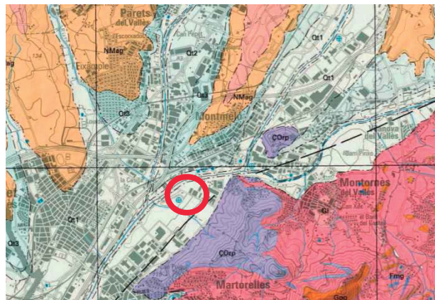
Imatge 4. Mapa Geològic (Font: Mapa geològic del Vallès Oriental )
