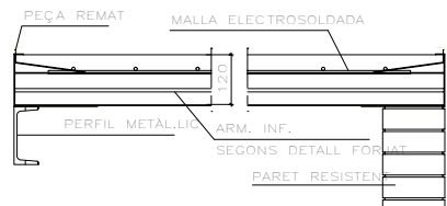
B4- DETALL RECOLZAMENT FINAL FORJAT
