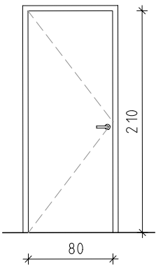
fi 2 Porta batent Fusta per pintar Color a decidir Pany i clau mastrejats P. Segona - 1 Unitat
