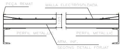
B3- DETALL RECOLZAMENT FINAL FORJAT
