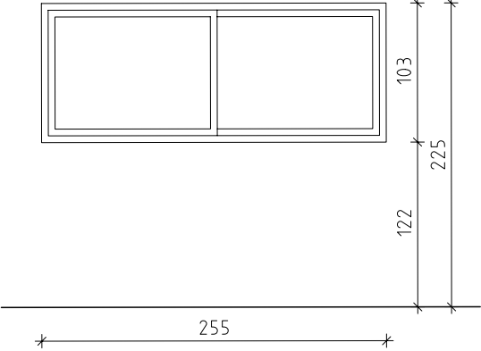
fe 3 Fusteria de PVC 2 fulles correderes 4+4/10/6+6 baix emisiu interior Color Blanc Uh<2,10 w/m²k Permeabilitat a l'aire Classe 3 (≤ 9 m³/hm²) P. Baixa - 1 Unit
