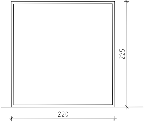
fe 2 Fusteria de PVC 1fulla ixè 4+4/10/6+6 baix emisiu interior Color Blanc Uh<2,10 w/m²k Permeabilitat a l'aire Classe 3 (≤ 9 m³/hm²) P. Baixa - 1 Unit
