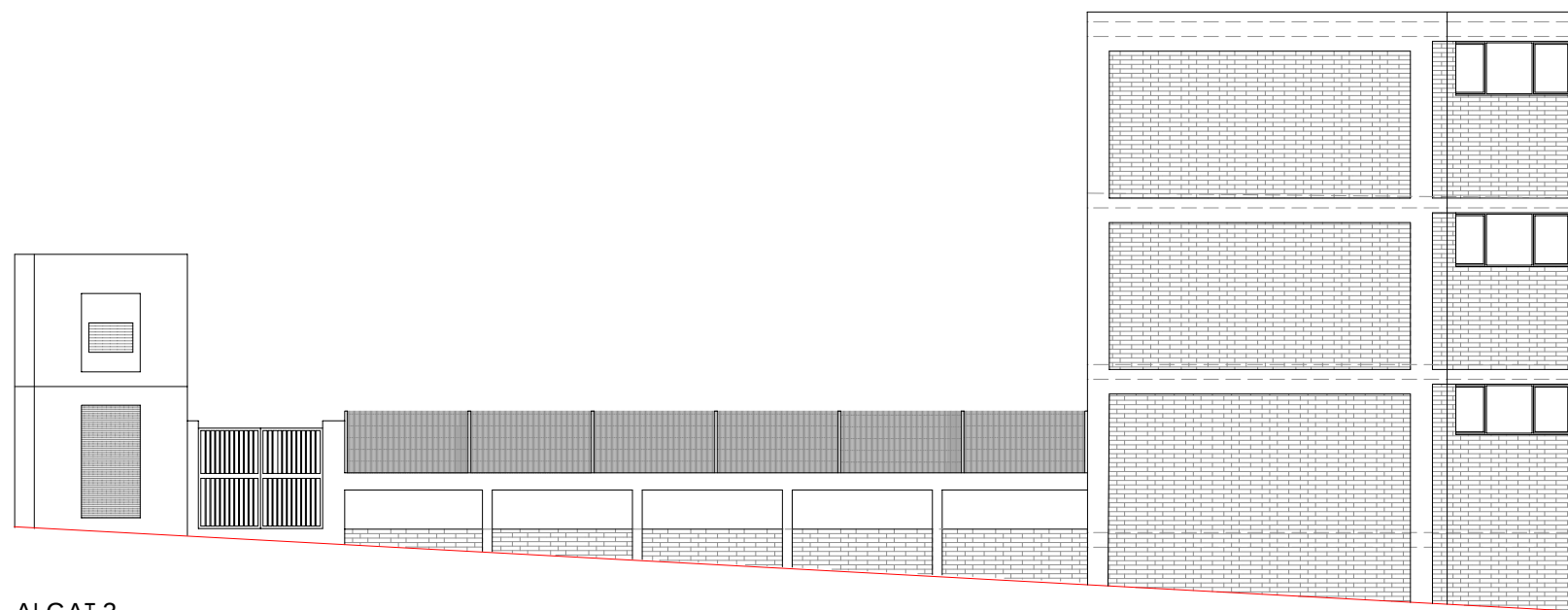
ALÇAT 3
