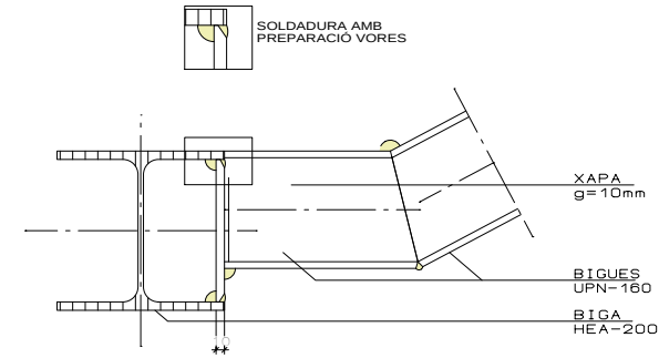
A3- UNIO ARRENCADA BRANCAL AMB BIGA METÀL·LICA UNIO ARTICULADA
