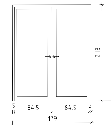
fe 1 Fusteria de PVC 2 fulles batents 4+4/10/6+6 baix emisiu interior Color Blanc Pany i clau mastrejats Uh<2,10 w/m²k Permeabilitat a l'aire Classe 3 (≤ 9 m³/hm²) P. Baixa - 1 Unit
