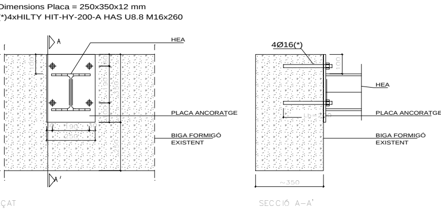
B2- RECOLZAMENT EN BIGA DE FORMIGÓ
