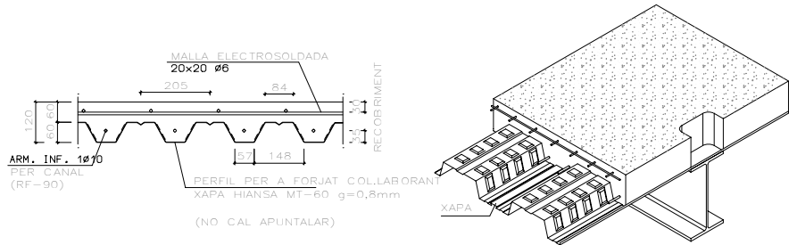
H1- SECCIÓ TIPUS FORJAT XAPA COL·LABORANT MT-60
