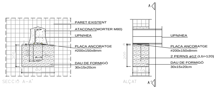
B1- RECOLZAMENT EN PARET DE CÀRREGA
