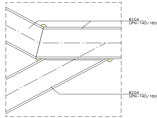
A4- BRANCAL ARRENCADA I ARRIBADA ESCALA UNIO RÍGIDA
