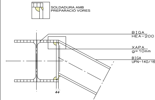
A2- UNIO ARRIBADA BRANCAL AMB BIGA METÀL·LICA UNIO ARTICULADA
