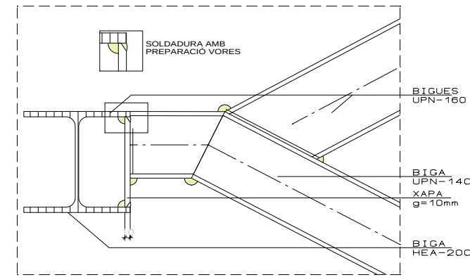
A5- UNIO BRANCAL ARRIBADA I ARRENCADA AMB BIGA METÀL·LICA RECOLZAMENT ARTICULAT
