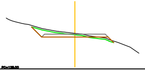
2=135.842 2=134.871 2=134.801 P.K.= 0+003.000 - Perfil N. 4
