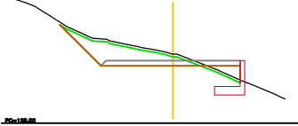
2=135.712 2=134.887 2=134.417 P.K.= 0+008.000 - Perfil N. 9
