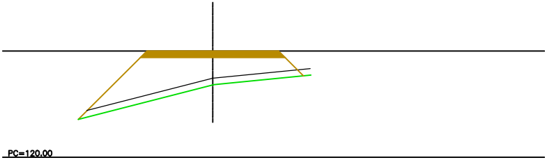
P.K.= 0+010.000 – Perfil N. 2
