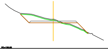
2=135.873 2=134.841 2=134.871 P.K.= 0+006.000 - Perfil N. 7
