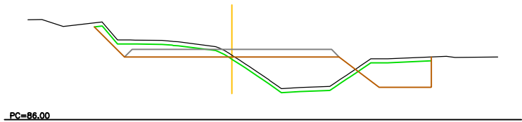
P.K.= 0+000.000 – Perfil N. 1
