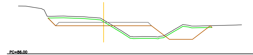
P.K.= 0+008.000 – Perfil N. 5
