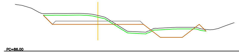
P.K.= 0+015.000 – Perfil N. 9
