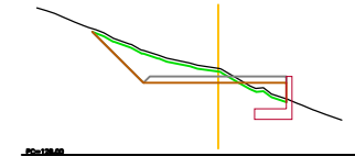
2=135.805 2=135.857 2=134.487 P.K.= 0+011.000 - Perfil N. 12
