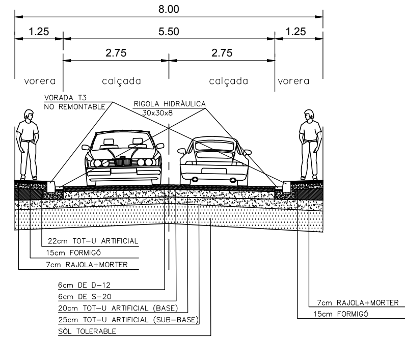
SECCIÓ B-B'
