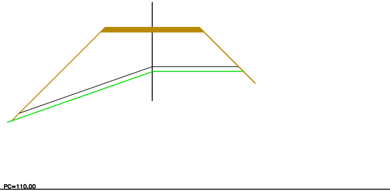
P.K.= 0+032.340 – Perfil N. 4
