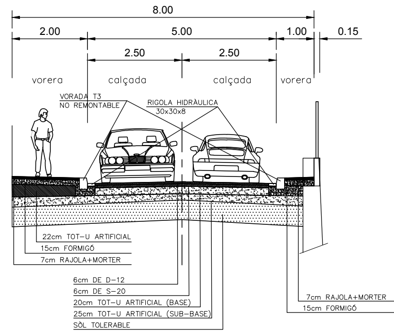
SECCIÓ A-A'
