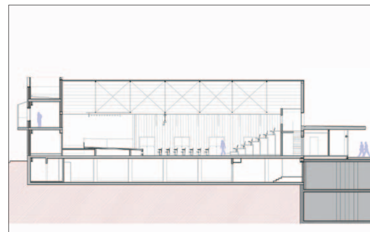
PLÀNOL DE SECCIÓ DE LA FAÇANA LATERAL
