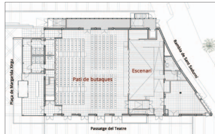
PLÀNOL DE LA PLANTA BAIXA
