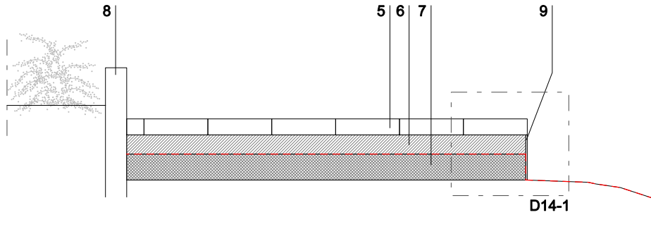
Secció A 1:50
