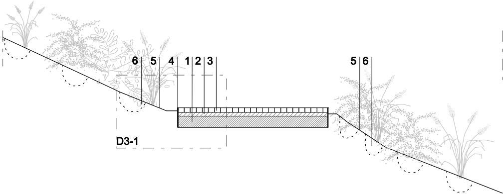
Secció 1/50
