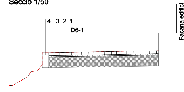
Secció 1/50
