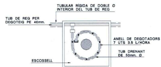
DETTALL PLANTA
