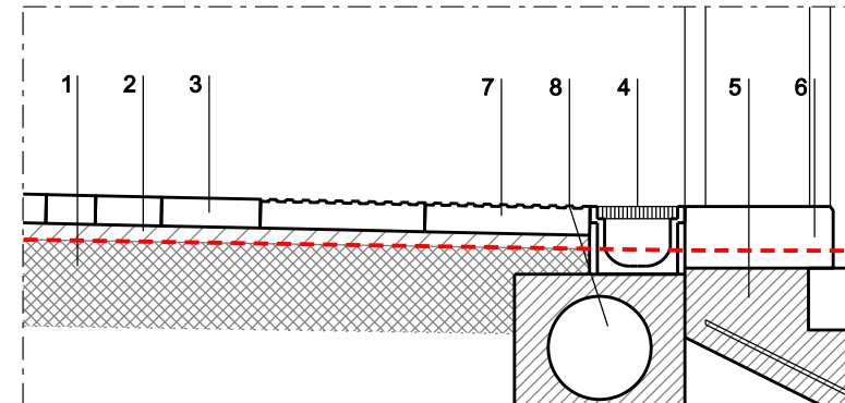
Detall D8-1 1/20
