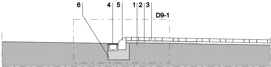
Secció 1/50
