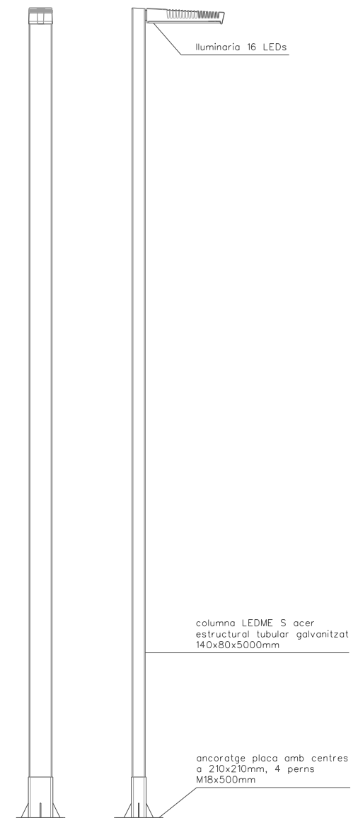
Alçats Il·luminària LEDME S LED
