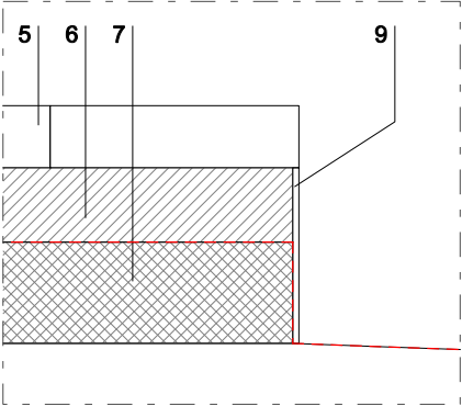
Detall D14-1 1/20
