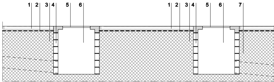
Secció. Pous 2 i 3
