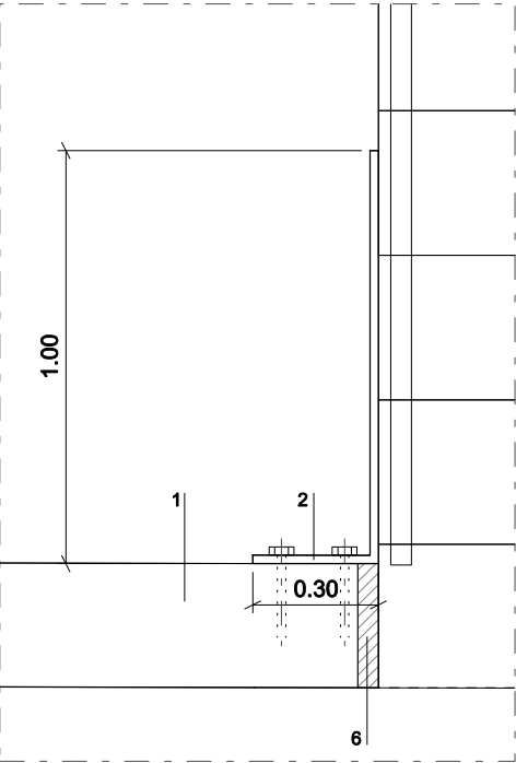
Detall D13-1 1/20
