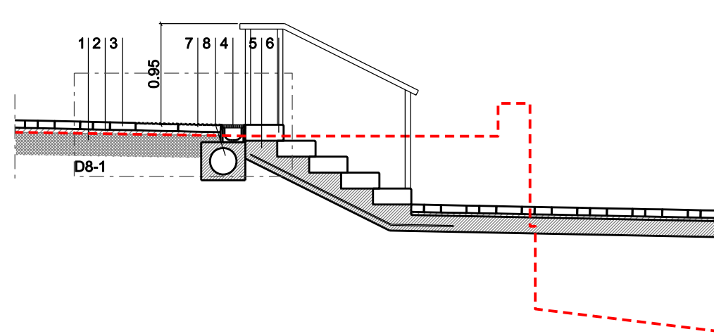
Secció 1/50
