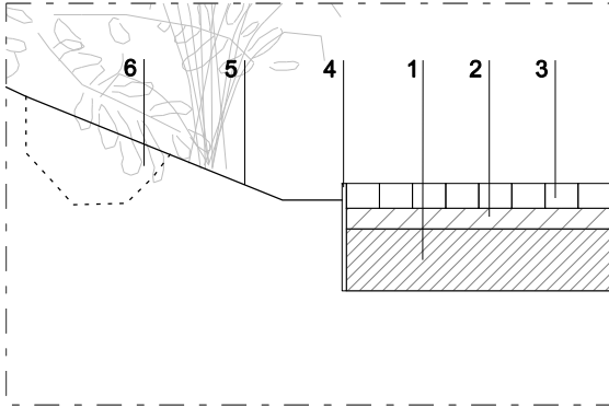
Detall D3-1 1/20
