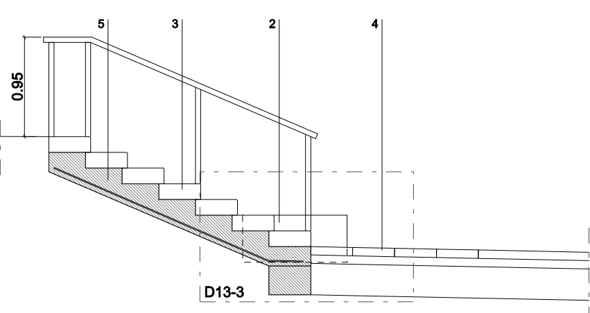
Secció A 1:50 (veure detall constructiu D12)
