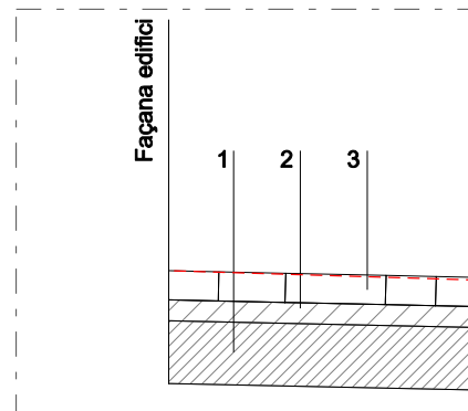
Detall D5-1 1/20
