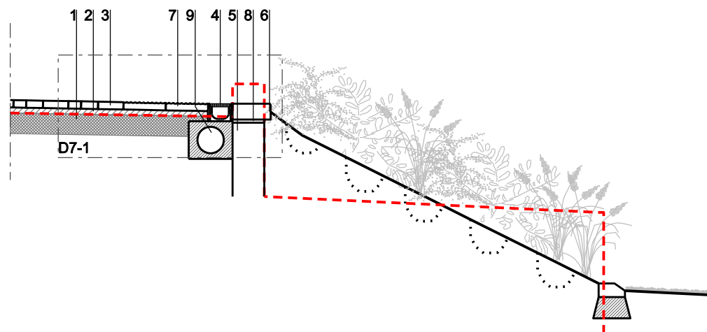
Secció 1/50
