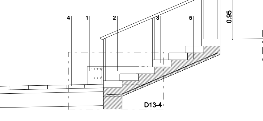
Secció B 1/50
