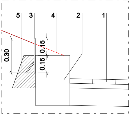
Detall D11-1 1/20
