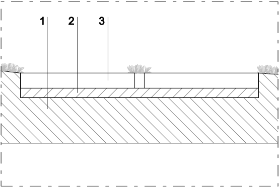
Detall D4-1 1/20
