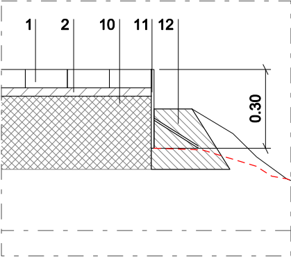
Detall D14-2 1/20
