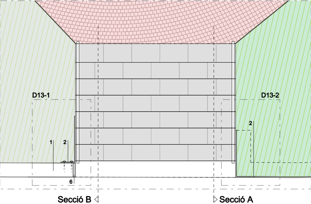
Planta 1/50
