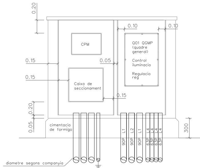
Detall quadre elèctric
