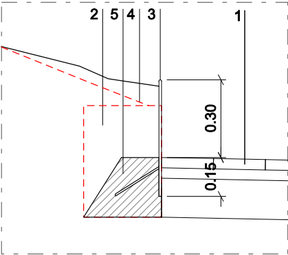
Detall D12-1 1/20
