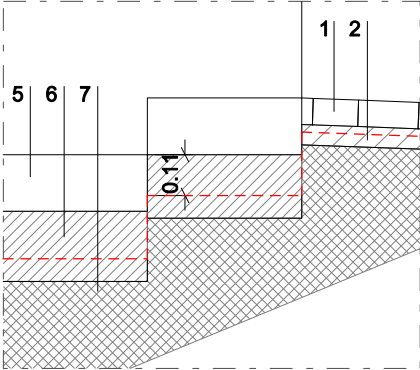
Detall D14-3 1/20
