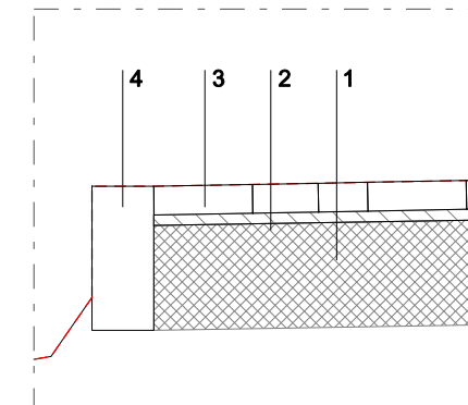
Detall D6-1 1/20
