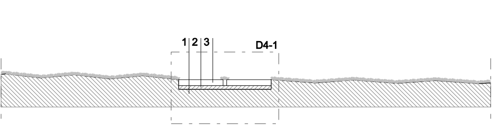
Secció 1/50
