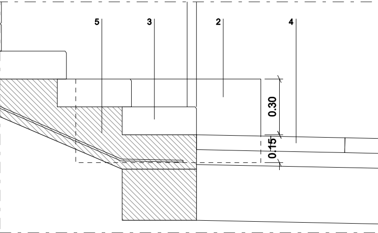
Detall D13-3 1/20
