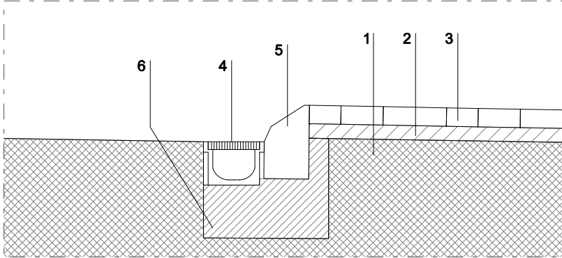
Detall D9-1 1/20
