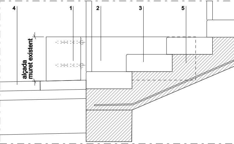
Detall D13-4 1/20
