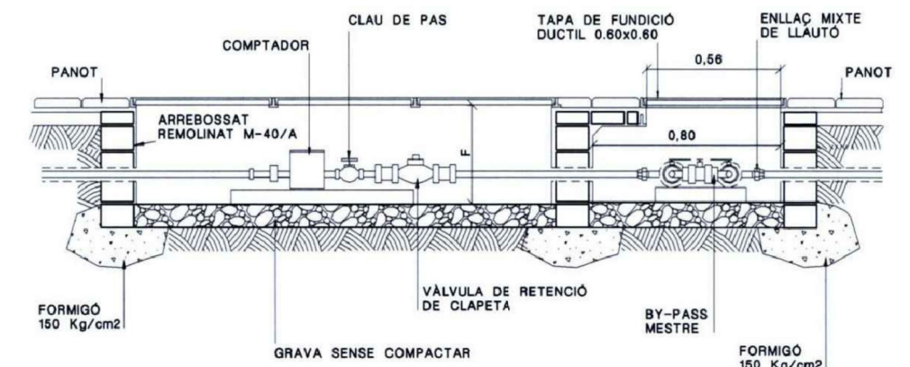
SECCIÓ
