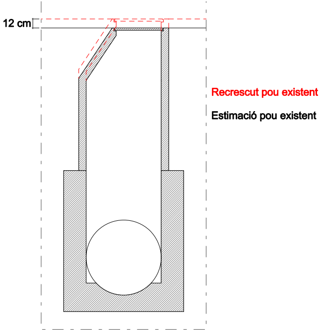
Secció
