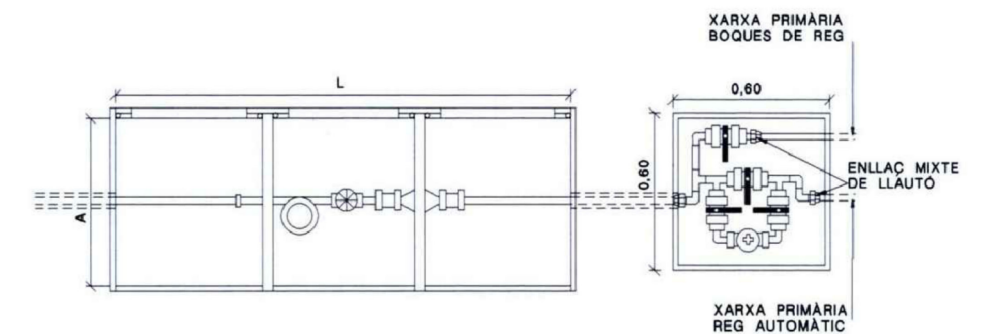
PLANTA
