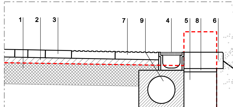
Detall D7-1 1/20
