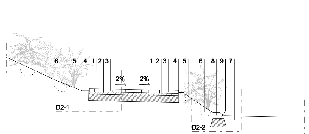
Secció 1/50
