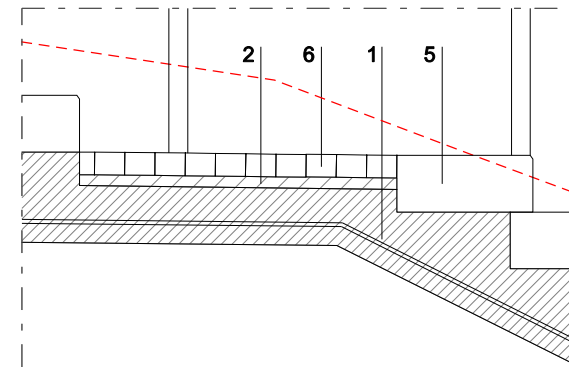
Detall D1-2 1/20
