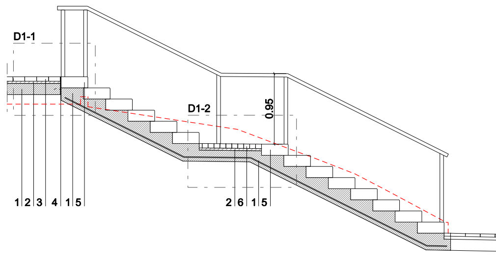
Secció 1/50
