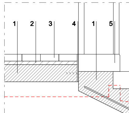
Detall D1-1 1/20
