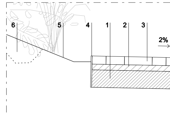
Detall D2-1 1/20
