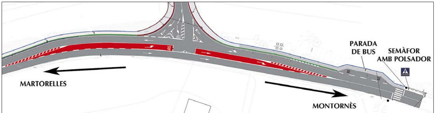
PLÀNOL DEL PROJECTE D'OBRES
